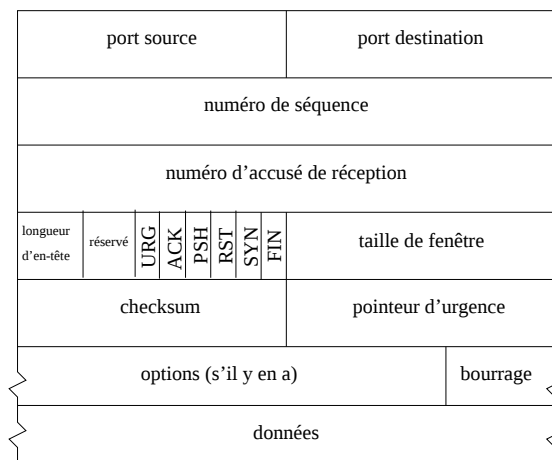
FIG. 2.25 - Format du segment TCP.
