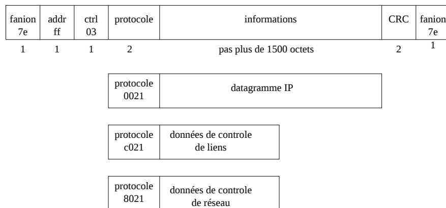
FIG. 2.14 - Encapsulation PPP.
