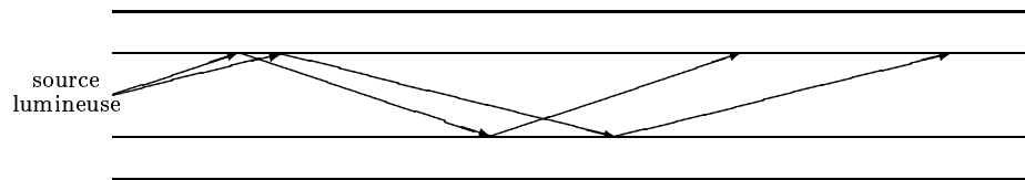
FIG. 1.11 - Réflexion interne.
