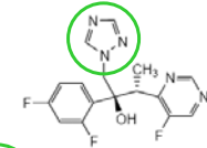
Voriconazole
