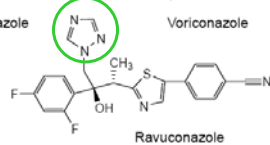
Ravuconazole
