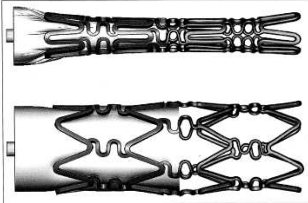
a Figure 1. La simulation sur ordinateur de l'expansion d'un stent (gauche) correspond nettement avec une expérience physique, très précisément mise en images par \mu CT (droite).
