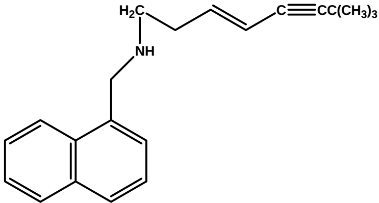
terbinafine
