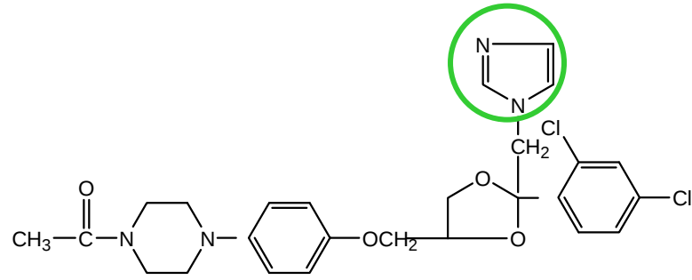
Ketoconazole
