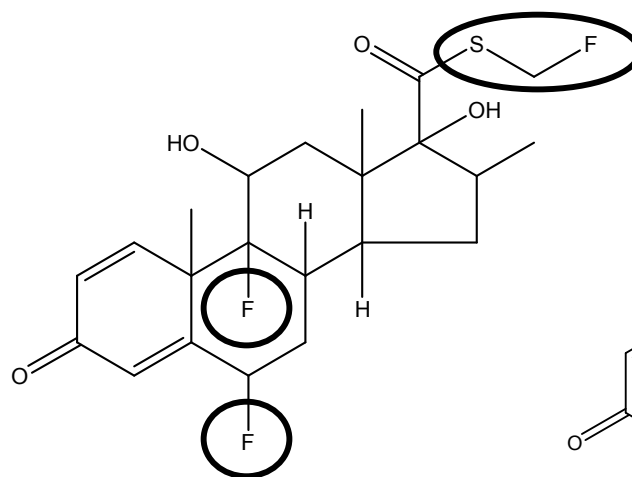
fluticasone
