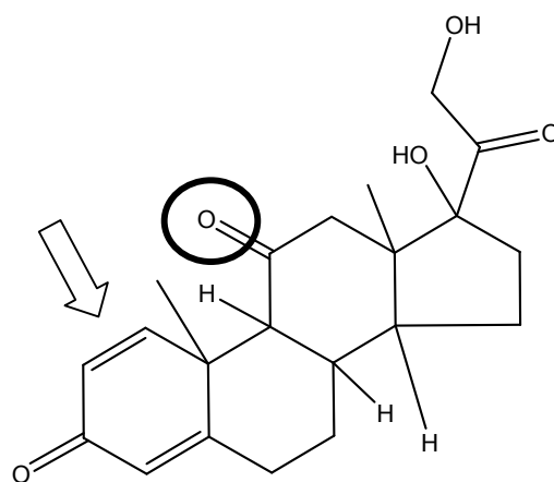
prednisone
