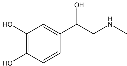
adrenaline
