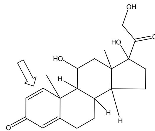
prednisolone
