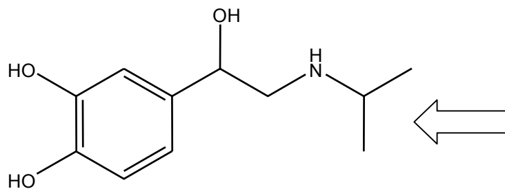
isoprénaline
