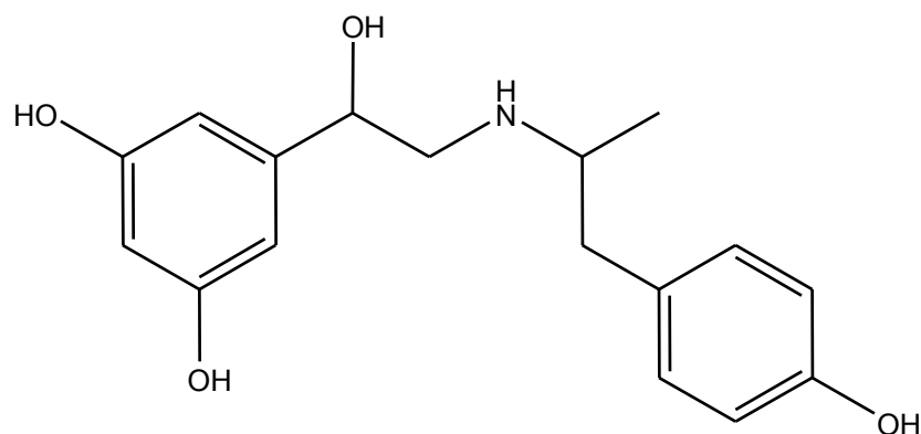
fénotérol
