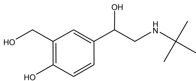
salbutamol
