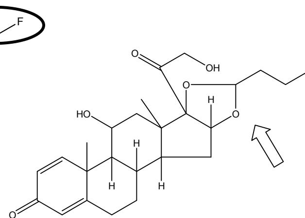
budénoside
