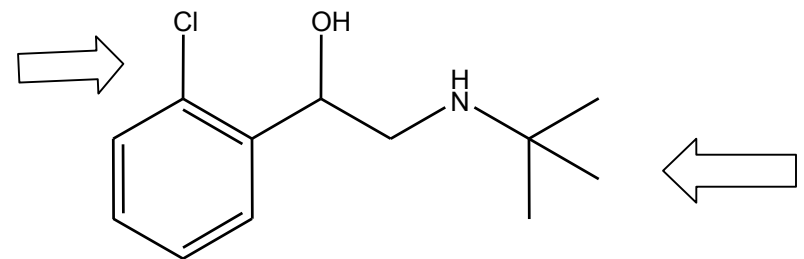
tulobuterol
