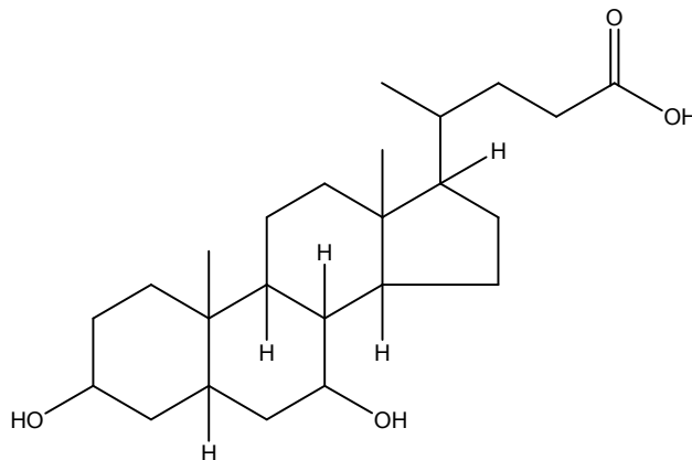
acide chénodésoxycholique
