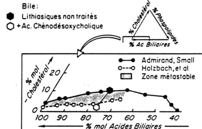
Fig. 2. Limites de solubilité du cholestérol dans la bile. Les points blancs et la ligne pointillée limitent la zone micellaire vraie : le cholestérol est toujours en solution. La zone hachurée est la zone métastable : le cholestérol, initialement en solution, précipite au bout de plusieurs heures. Au-dessus de la ligne limitée par les points noirs et la ligne continue, le cholestérol précipite habituellement immédiatement. L'hexagone noir représente la composition moyenne de la bile de sujets lithiasiques non traités ; l'hexagone blanc représente la composition moyenne de la bile de patients traités par l'acide chénodésoxycholique.
