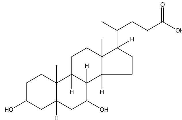
acide ursodésoxycholique
