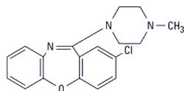
Loxapine
