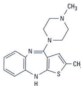
Olanzapine
