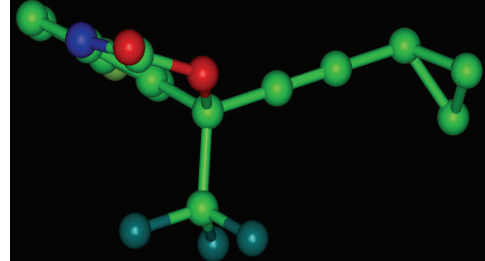
efavirenz
