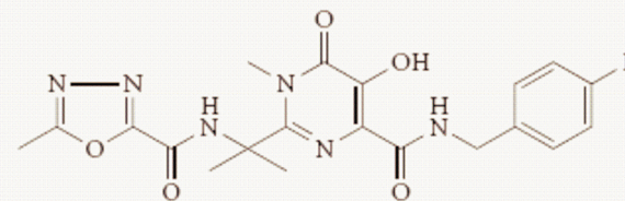
Raltegravir (MK-0518)
