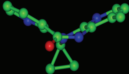
nevirapine
