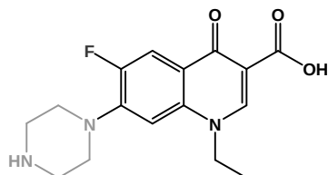
norfloxacin e
