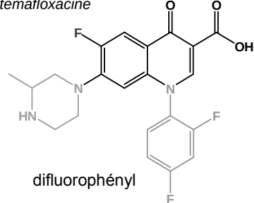
temafloxacin
