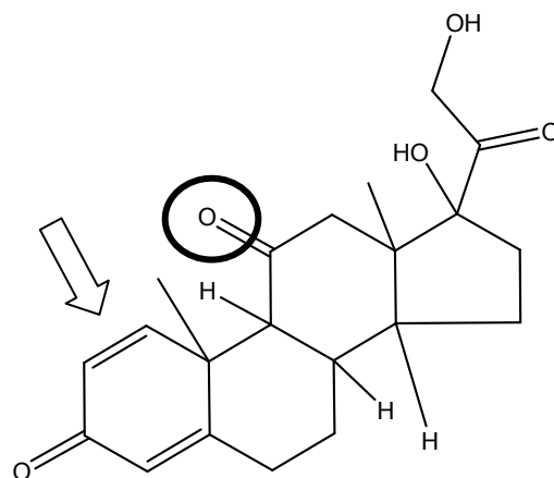
prednisone
