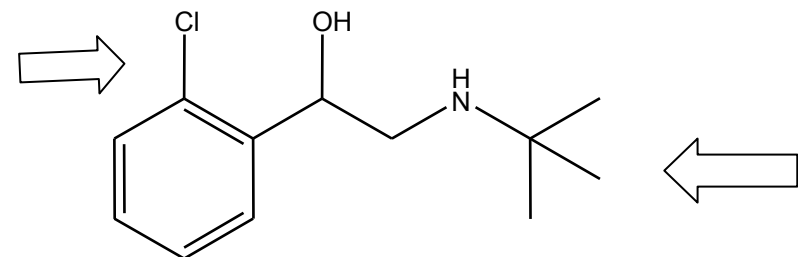
tulobuterol
