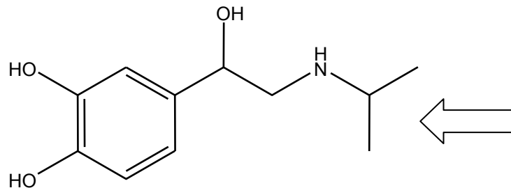
isoprénaline
