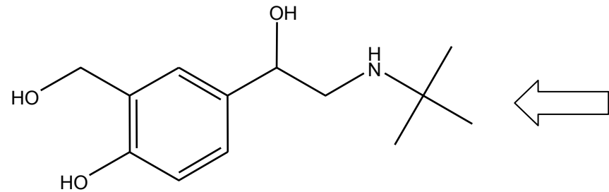
salbutamol
