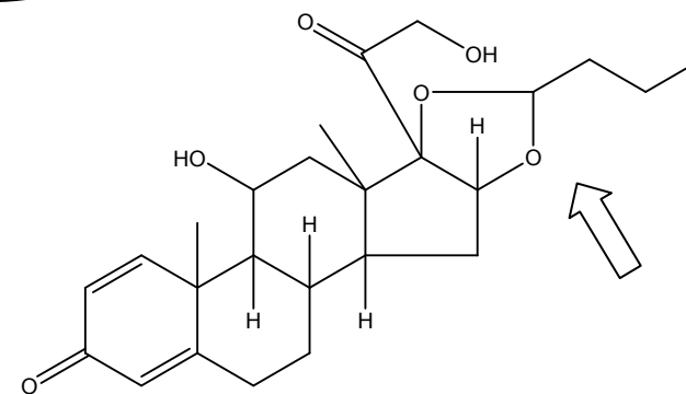
budénoside
