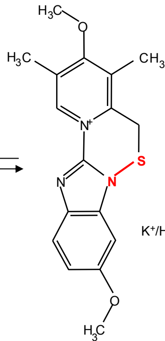
sulfénamide
