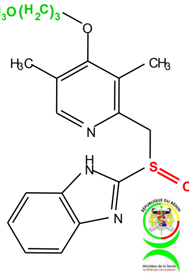
rabéprazole
