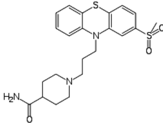
Metopimazine
