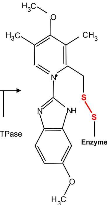
complexe enzyme-inhibiteur
