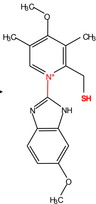
acide sulfénique
